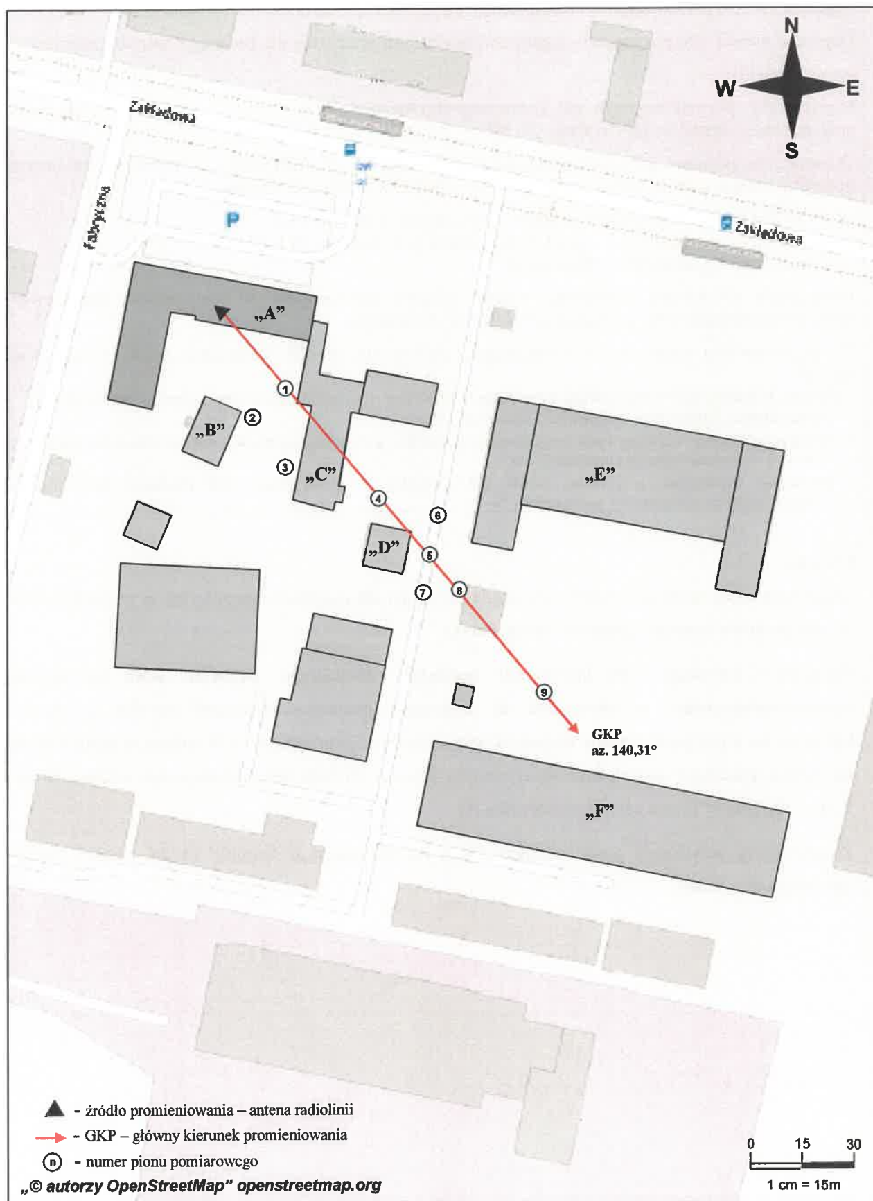
Rys. 1. Usytuowanie punktów i pionów pomiarowych w otoczeniu instalacji radiokomunikacyjnej Stacja Netia KONNB117-KONNM00020 Konin, ul. Zakładowa 7a
