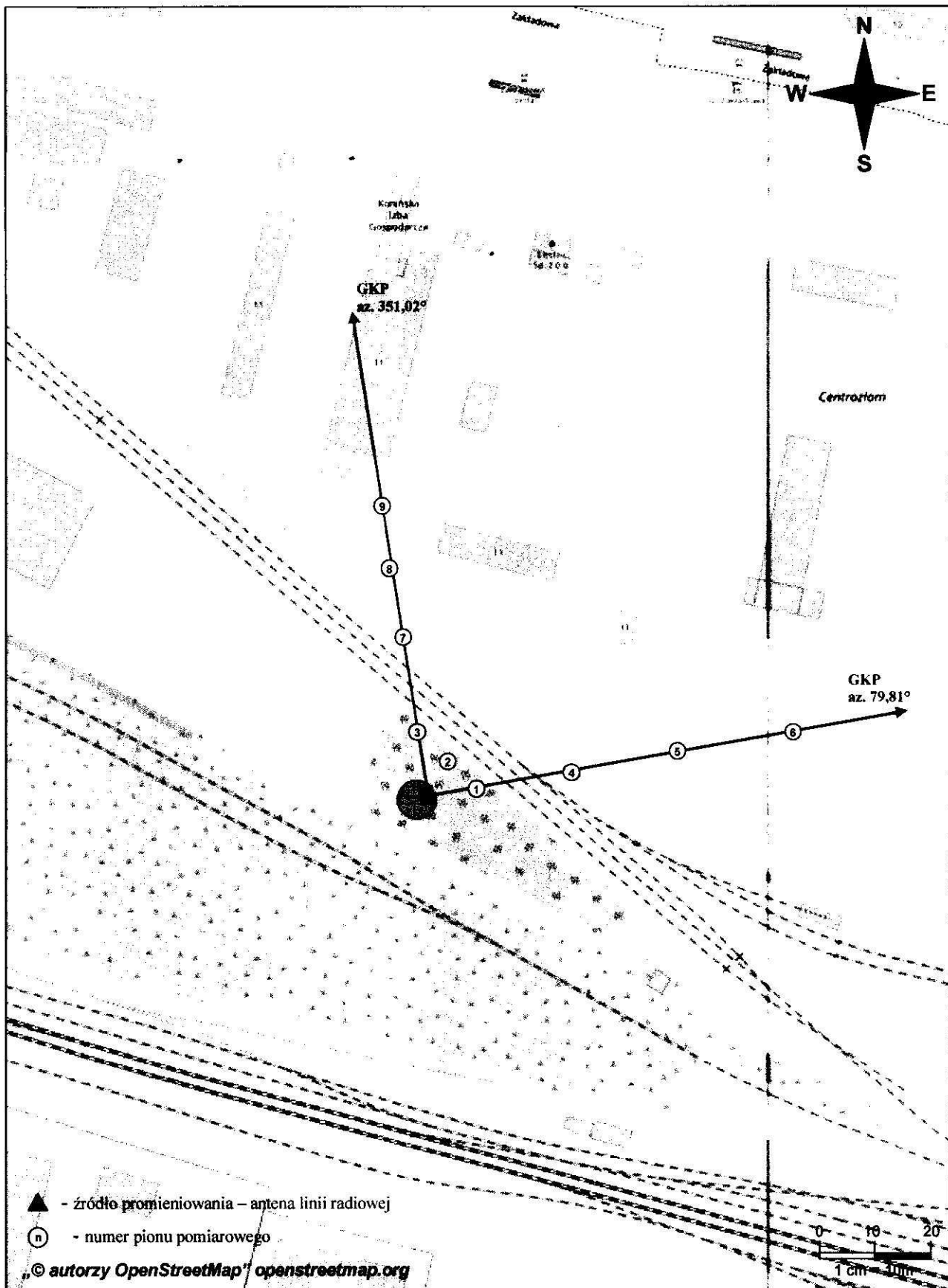
Rys. 1. Usytuowanie punktów i pionów pomiarowych w otoczeniu instalacji radiokomunikacyjnej Stacja Netia KONNB016-KONNM00003 Konin, ul. Parowozownia 1
