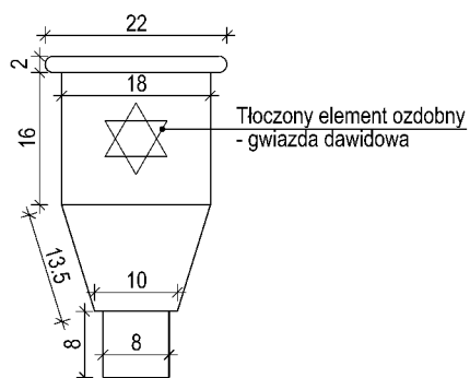
Kosz zlewowy - miedziany skala 1:10
