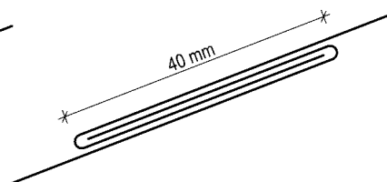
Przekrój podłużny przez łączy blach metodą zwyczajnego rąbka poprzecznego dla połaci o nachyleniu min 7°
