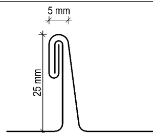
Przekrój poprzeczny przez łączy blach metodą rąbka stojącego podwójnego dla połaci o nachyleniu min. 3°
