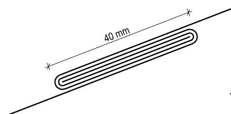
Przekrój podłużny przez łączy blach metodą podwójnego rąbka poprzecznego dla połaci o nachyleniu min 25°
