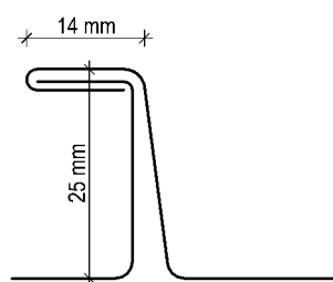
Przekrój poprzeczny przez łączy blach metodą rąbka kąowego stojącego dla połaci o nachyleniu większym niż 25°
